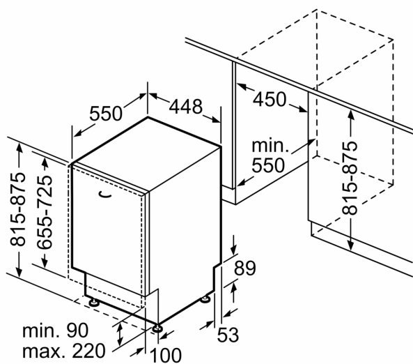
Méretek mm-ben
