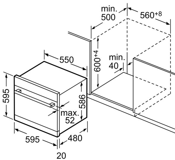
Méretetek mm-ben
