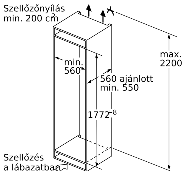
Méretetek mm-be
