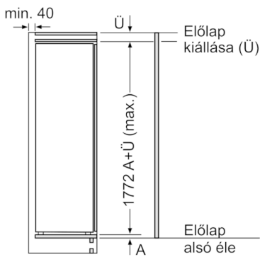
Méretetek mm-ben
