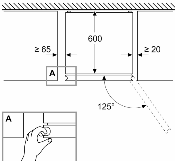
Méretetek mm-ben
