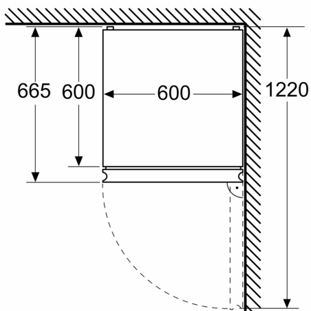
Méretetek mm-ben
