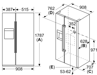
Méretetek mm-ben
