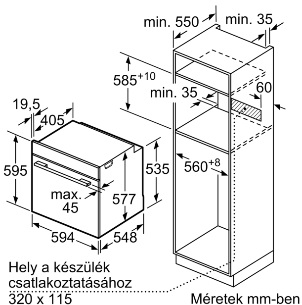
Méretetek mm-ben
