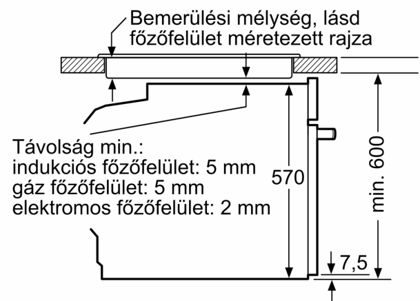
Méretek mm-ben
