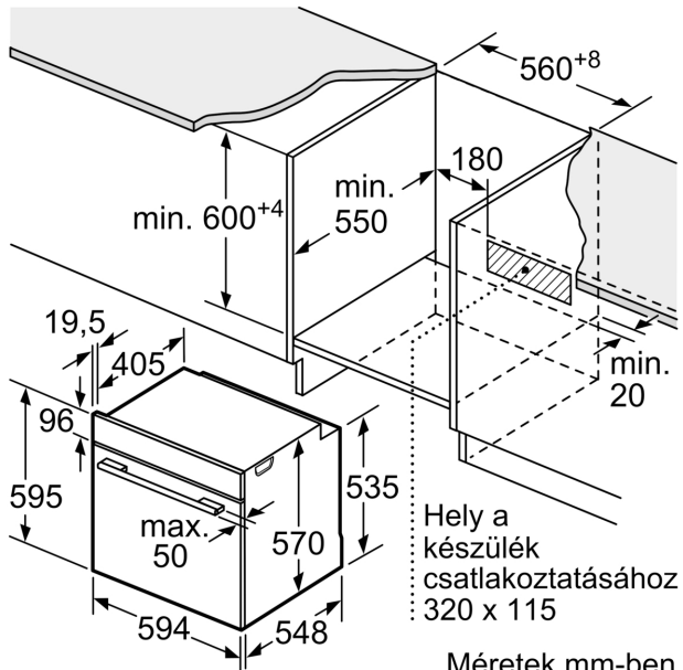
Méretek mm-ben
