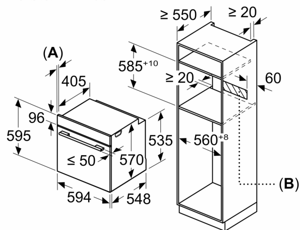
Méretetek mm-ben
