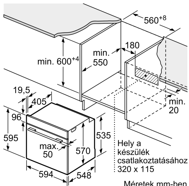
Méretetek mm-ben
