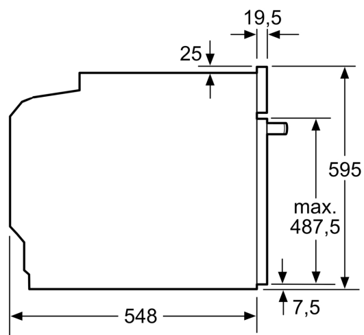
Méretetek mm-ben
