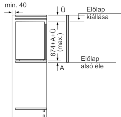
Méretetek mm-ben
