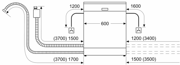
מידות במ"מ
