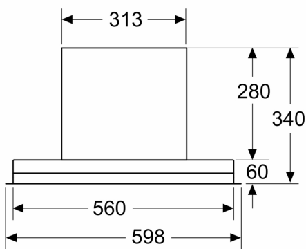
Mesures en mm Vue de face
