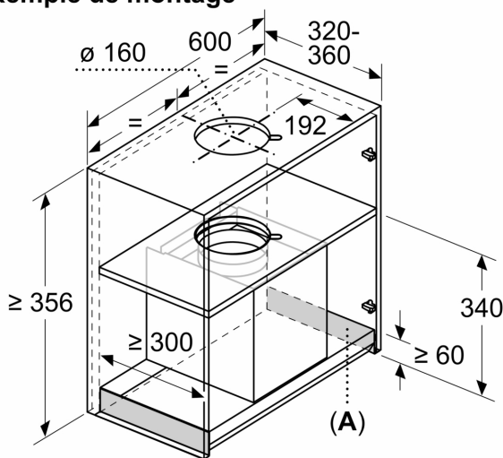
Mesures en mm Exemple de montage
