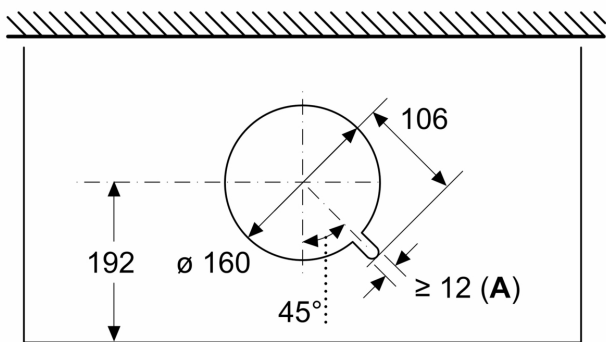
Mesures en mm Vue du dessus
