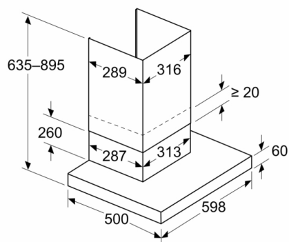
Mesures en mm Appareil en mode d'évacuation d'air
