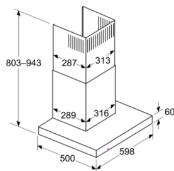
Mesures en mm Perspective du système de recyclage
