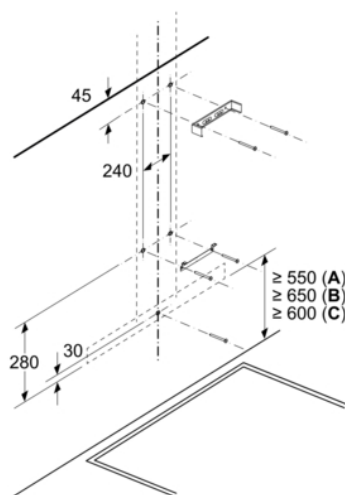
Mesures en mm Installation murale avec cheminée
