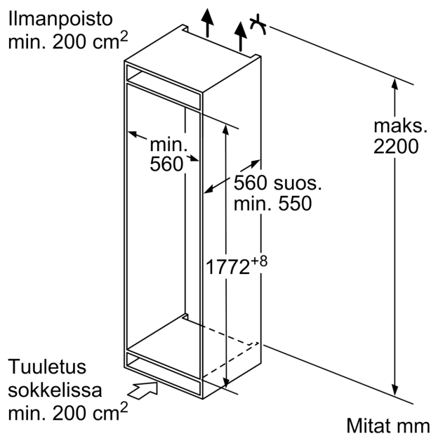
Mitat mm
