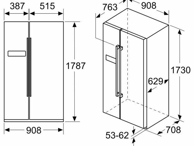
Mitat mm
