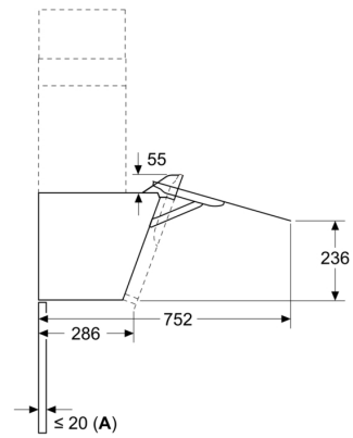
Mitat mm
