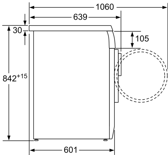
Mõõdud (mm)
