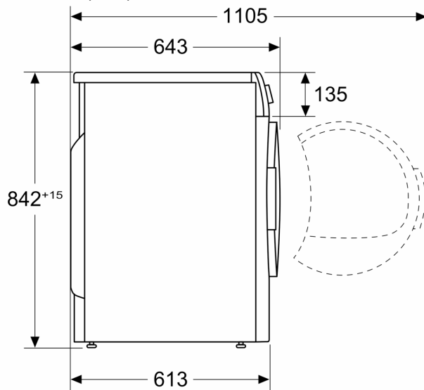
Mõõdud (mm)
