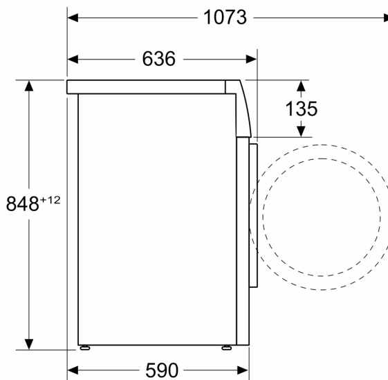
Mõõdud (mm)
