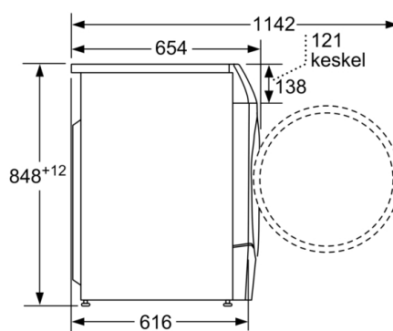
Mõõdud (mm)
