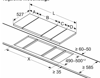
Mõõdud (mm) Pilt Domino kombinatsioonivõimaluste tabeli kohta koos vastavate seadmete väljalõike mõõtmetega
