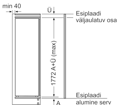
Mõõdud (mm)
