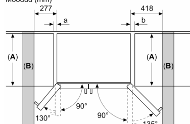
Mõõdud (mm)
