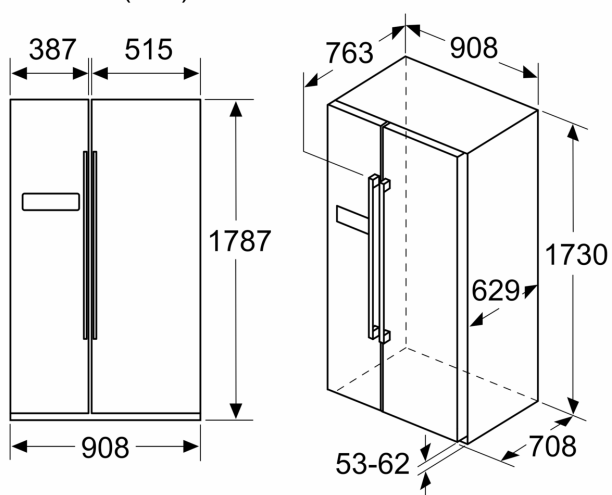
Mõõdud (mm)
