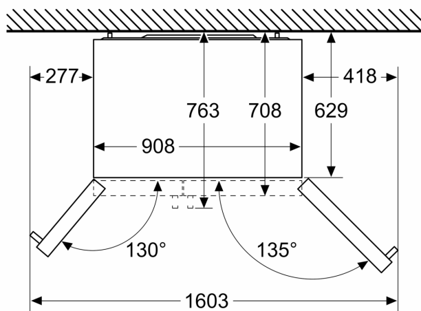
Mõõdud (mm)
