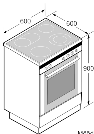
Mõõdud (mm)
