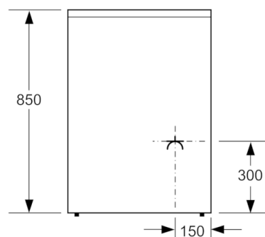
Mõõdud (mm)
