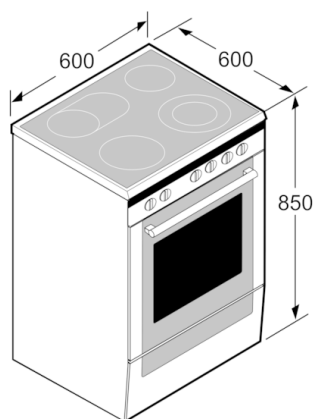
Mõõdud (mm)
