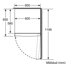
Mõõdud (mm)
