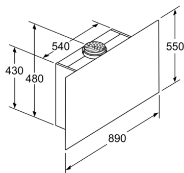
Seade tsirkulatsioonirežiimil ilma kanalita Vajalik on tsirkulatsioonikomplekt Mõõdud (mm)
