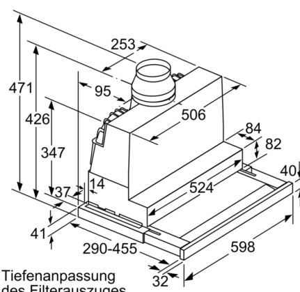
Mõõdud (mm)
