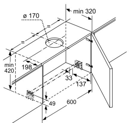
Mõõdud (mm)
