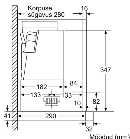
Mõõdud (mm)
