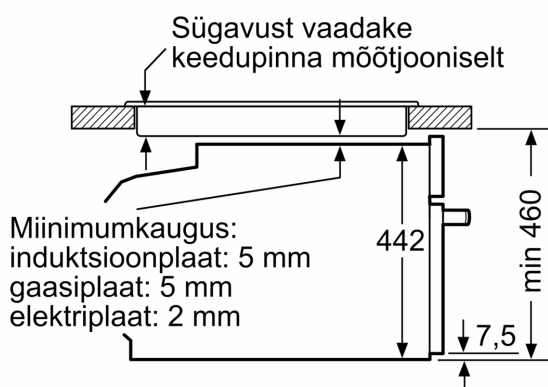
Mõõdud (mm)
