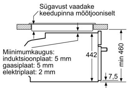
Mõõdud (mm)
