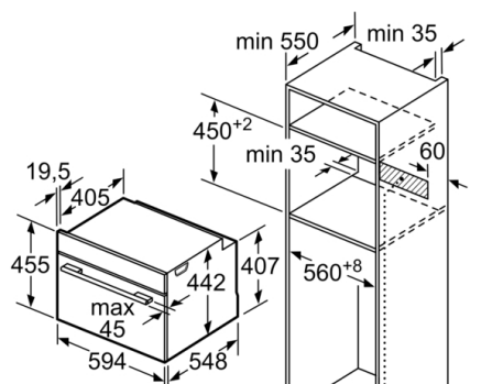
Mõõdud (mm)
