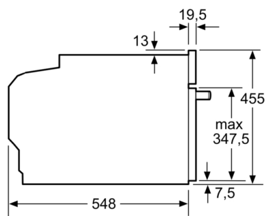
Mõõdud (mm)
