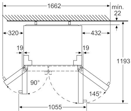
Cajones completamente extraíbles con un ángulo de apertura de la puerta de 145°. Dimensiones en mm
