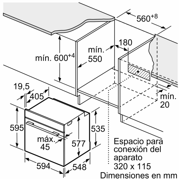
Espacio para conexión del aparato 320 x 115
