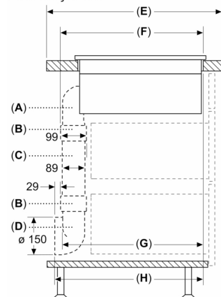
Διαστάσεις σε mm
