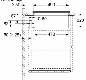
Διαστάσεις σε mm Πλάγια όψη
