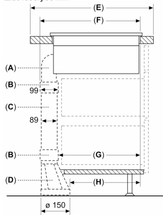
Διαστάσεις σε mm
