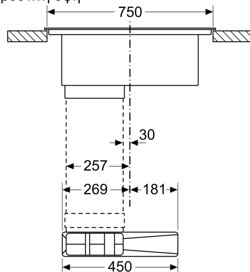
Διαστάσεις σε mm Μπροστινή όψη
