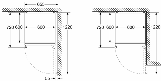
Διαστάσεις σε mm
