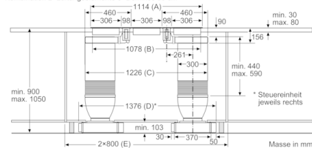
Kombination 2x Lüftungselemente 3x Dominos 30 cm
