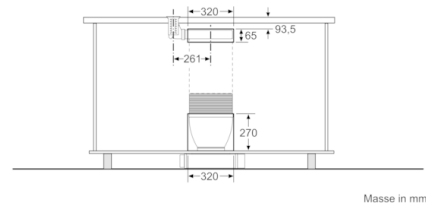
Ausschnitt in Rückwand
