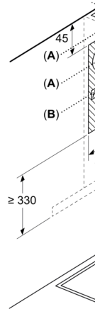
Maße in mm
