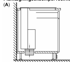
A: Ydervæg – U-værdi \leq 0,5 \text{ W/(m}^2\text{K)}
