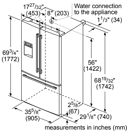
B26FT50SNS Dimensions
