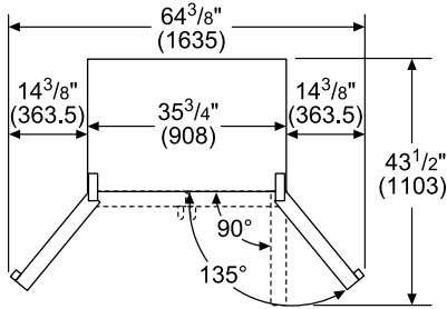
36" Freestanding Dimensions (Overhead Views)
