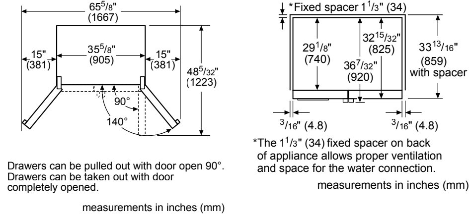
B26FT50SNS Dimensions (Overhead Views)
