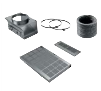
DWZ 0AK0S0: zestaw startowy do pracy w obiegu zamkniętym do regeneracji. Zawiera zwrotnicę do pracy w obiegu zamkniętym, filtr z aktywnym węglem do wielokrotnej regeneracji (2 sztuki), elastyczny wąż i materiał do mocowania
