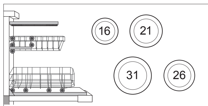
Systém košů s příborovou zásuvkou Vario u myček vysokých 81,5 cm
