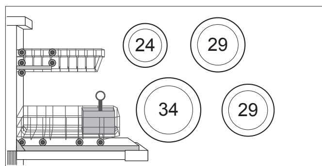
Systém košů bez příborové zásuvky Vario u myček vysokých 86,5 cm (o 5 cm vyšší myčka nádobí poskytuje prostor navíc pro vysoké nádobí v dolním koši)
