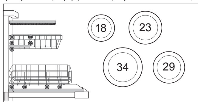
Systém košů s příborovou zásuvkou Vario u myček vysokých 86,5 cm (o 5 cm vyšší myčka nádobí poskytuje prostor navíc pro vysoké nádobí v dolním koši)
