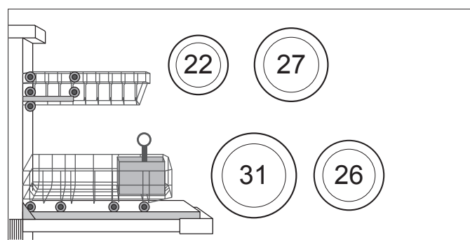
Systém košů bez příborové zásuvky Vario u myček vysokých 81,5 cm
