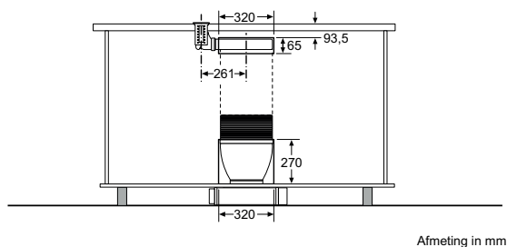
Uitsparing in achterwand
