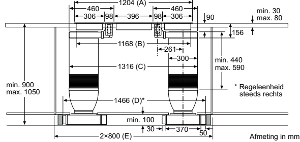
Combinatie 2×Ventilatie-elementen 2×Dominos 30 cm 1×Domino 40 cm
