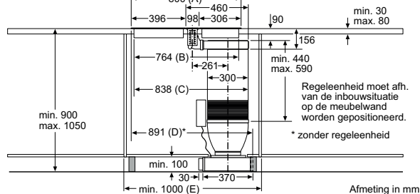
Combinatie 1×Ventilatie-element 1×Domino 30 cm 1×Domino 40 cm
