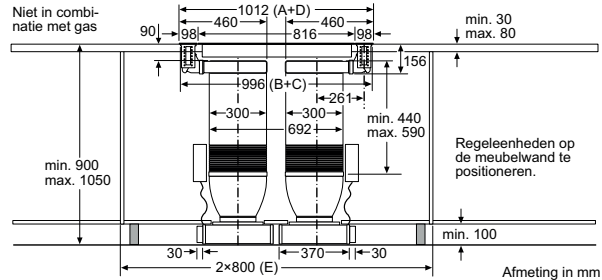
Combinatie 2×Ventilatie-elementen 1×Kookzone 80 cm
