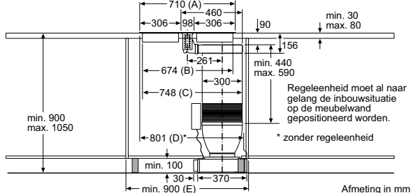
Combinatie 1×Ventilatie-element 2×Dominos 30 cm
