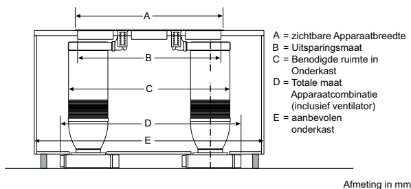
Combinatie 2×Ventilatie-elementen 3×Dominos 30 cm
