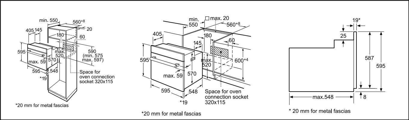
HBN411E2K, HBN331E1K, HBA23B251K
