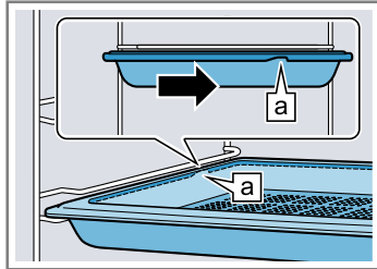
Panier va-peur perforé, taille XL
