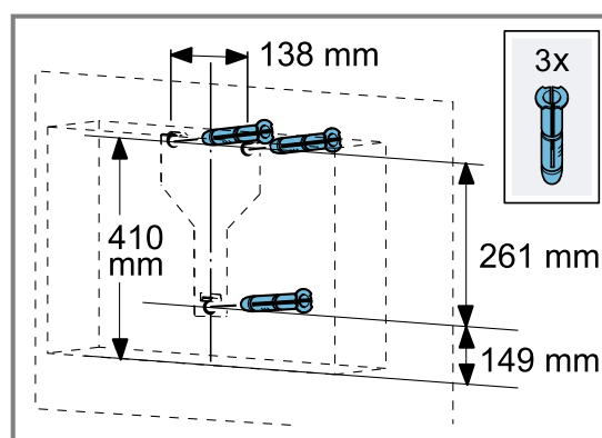
Wariant A: Płaski okap kuchenny bez obudowy kominowej
