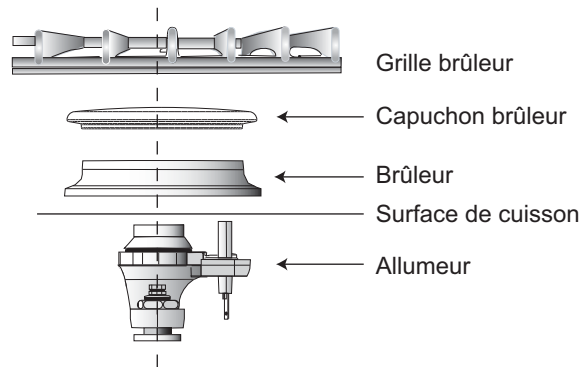
Figure 1: Grille côté droit - vue latérale
