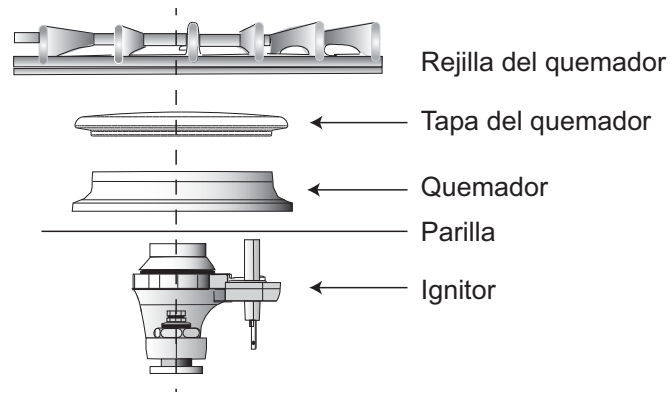
Figura 1: Quemador Lado Derecho - Vista Lateral
