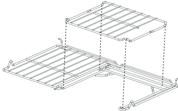
Figura 7: Rejilla media del horno
