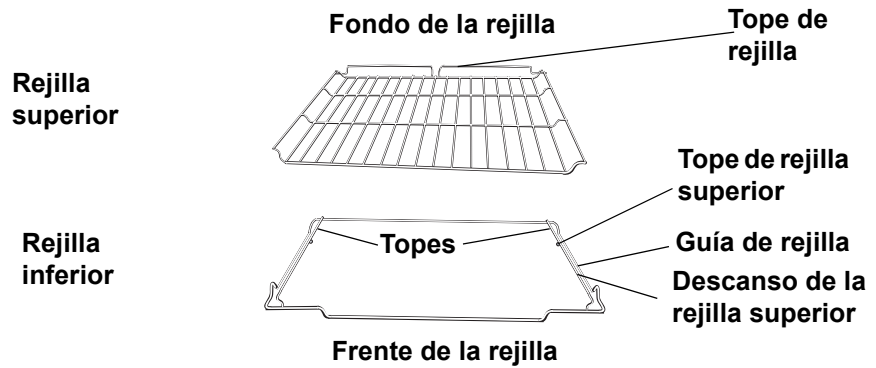
Figura 3: Rejilla de extensión completa
