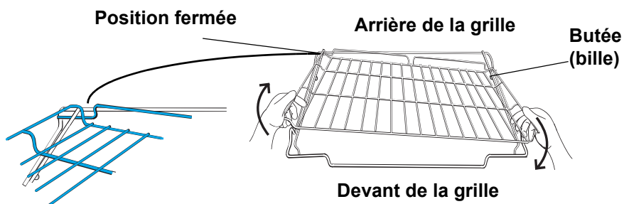
Figure 6: Démontage
