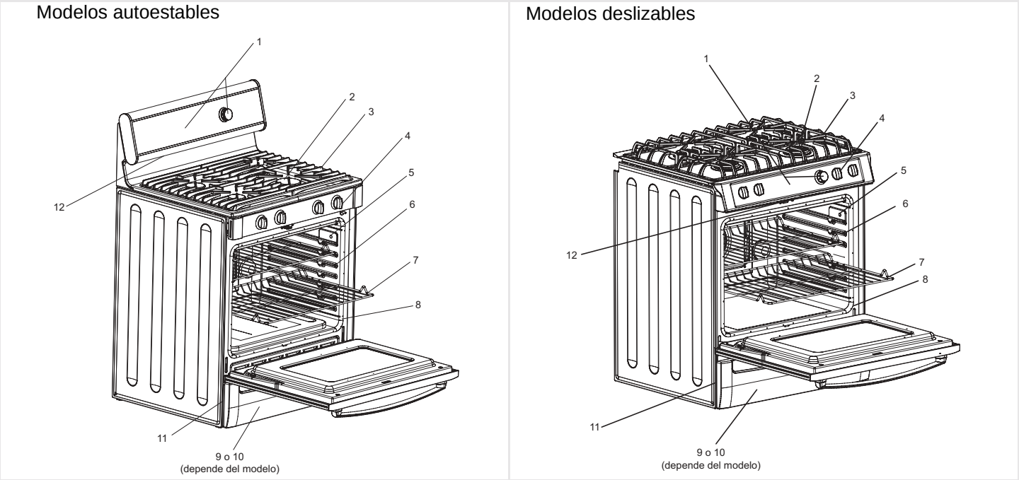
Figura 2: Partes y Accesorios
