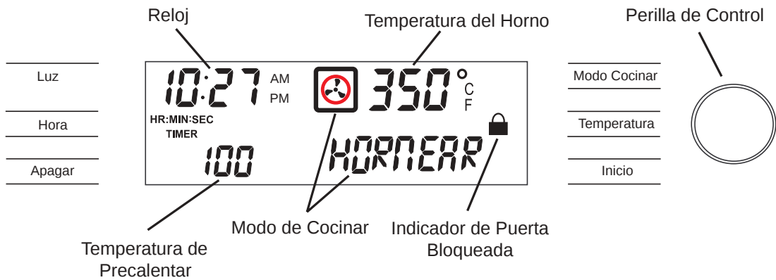
Figura 13:Panel de control del horno
