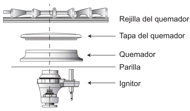
Figura 3: Quemador Lado Derecho - Vista Lateral
