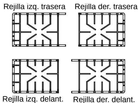
Figura 5: Rejillas para modelos empotrables - Vista superior
