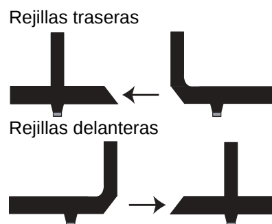
Figura 6: Instalar rejillas para modelos empotrables - Vista lateral
