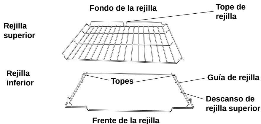
Figura 8: Rejilla de extensión completa
