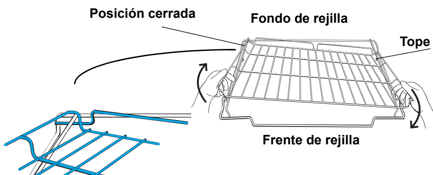
Figura 6: Desmontaje
