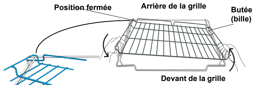
Figure 7: Réassemblage
