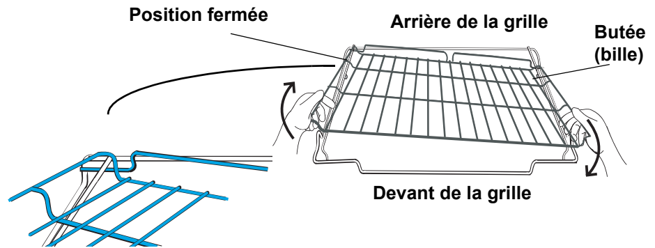
Figure 4: Démontage
