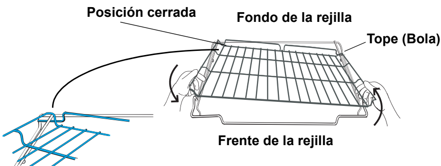
Figura 5: Reensamblado
